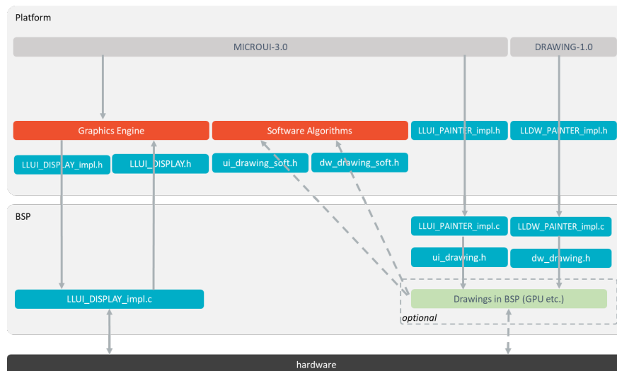
Fig. 42: Display Low Level API
