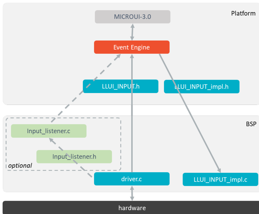
Fig. 40: Input Low Level API
