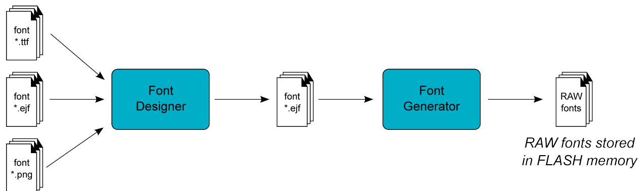
Fig. 44: Font Generation
