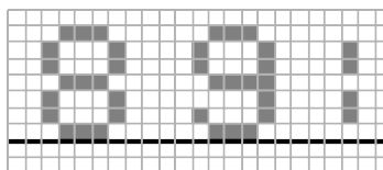
Fig. 46: Font baseline
