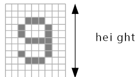
Fig. 45: Font Height
