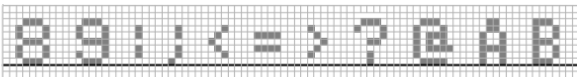
Fig. 72: The Baseline
