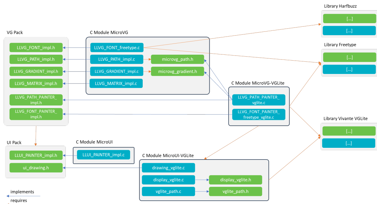
Fig. 62: MicroVG C Modules
