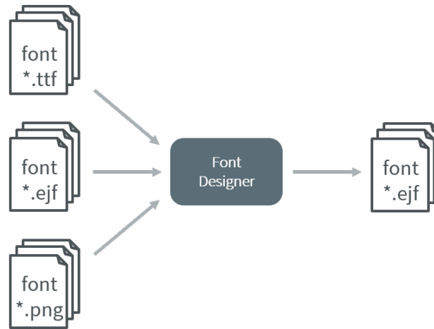
Fig. 71: Font Generation
