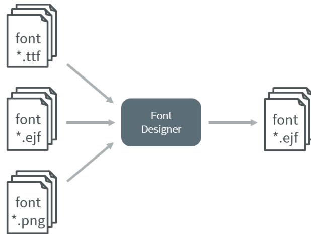
Fig. 75: Font Generation
