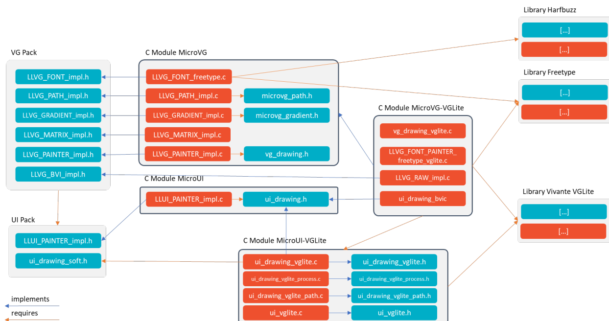
Fig. 65: MicroVG C Modules
