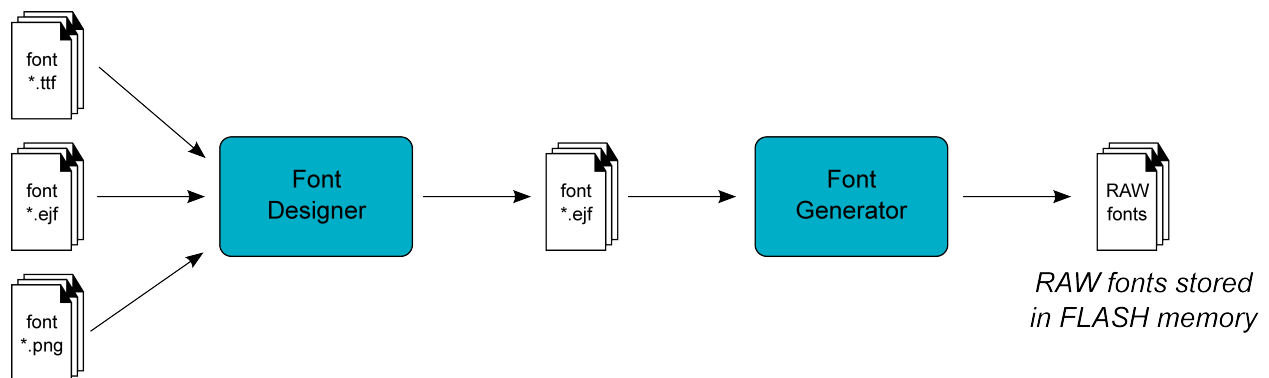
Fig. 42: Font Generation
