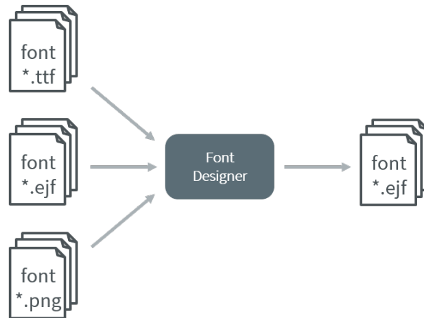
Fig. 61: Font Generation
