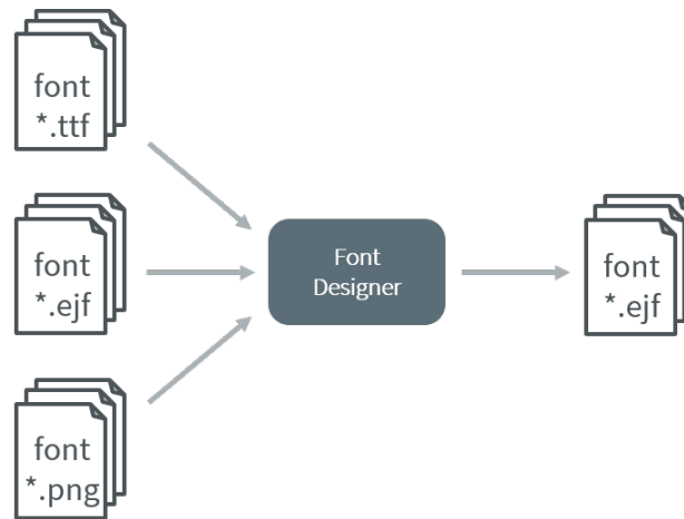
Fig. 30: Font Generation
