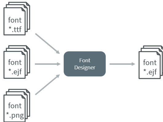
Fig. 54: Font Generation
