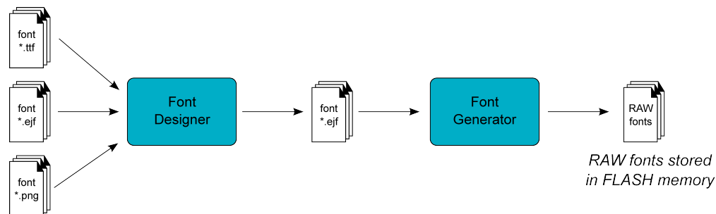
Fig. 38: Font Generation
