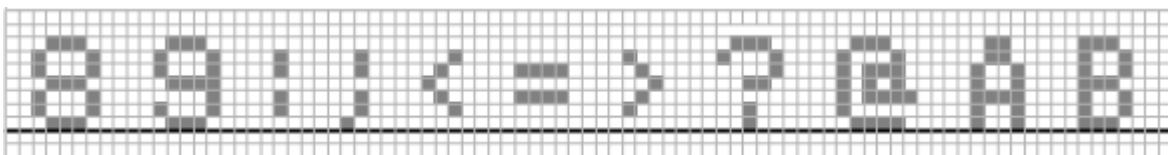
Fig. 56: The Baseline
