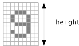
Fig. 39: Font Height
