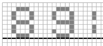
Fig. 40: Font baseline
