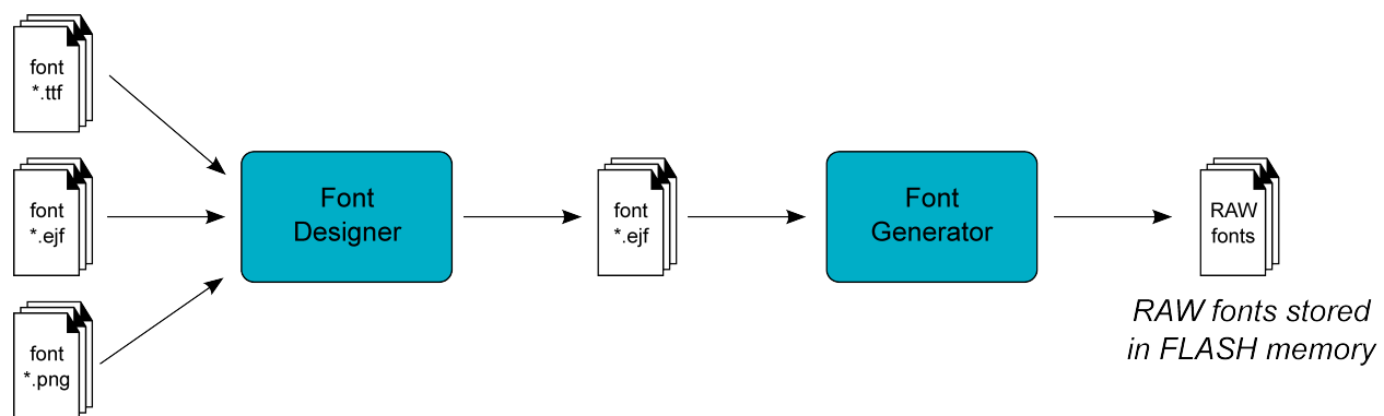
Fig. 38: Font Generation
