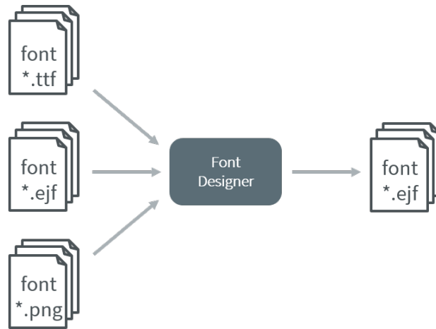
Fig. 56: Font Generation
